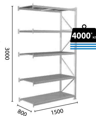
MS Pro 300/150x80/5
