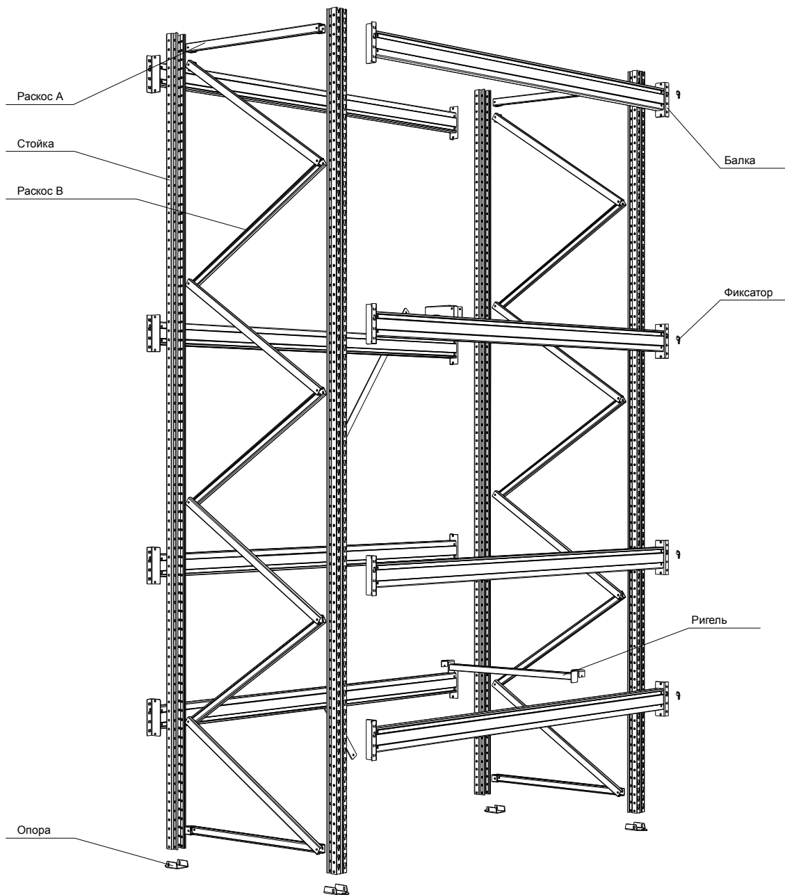
Схема сборки фронтального складского стеллажа
